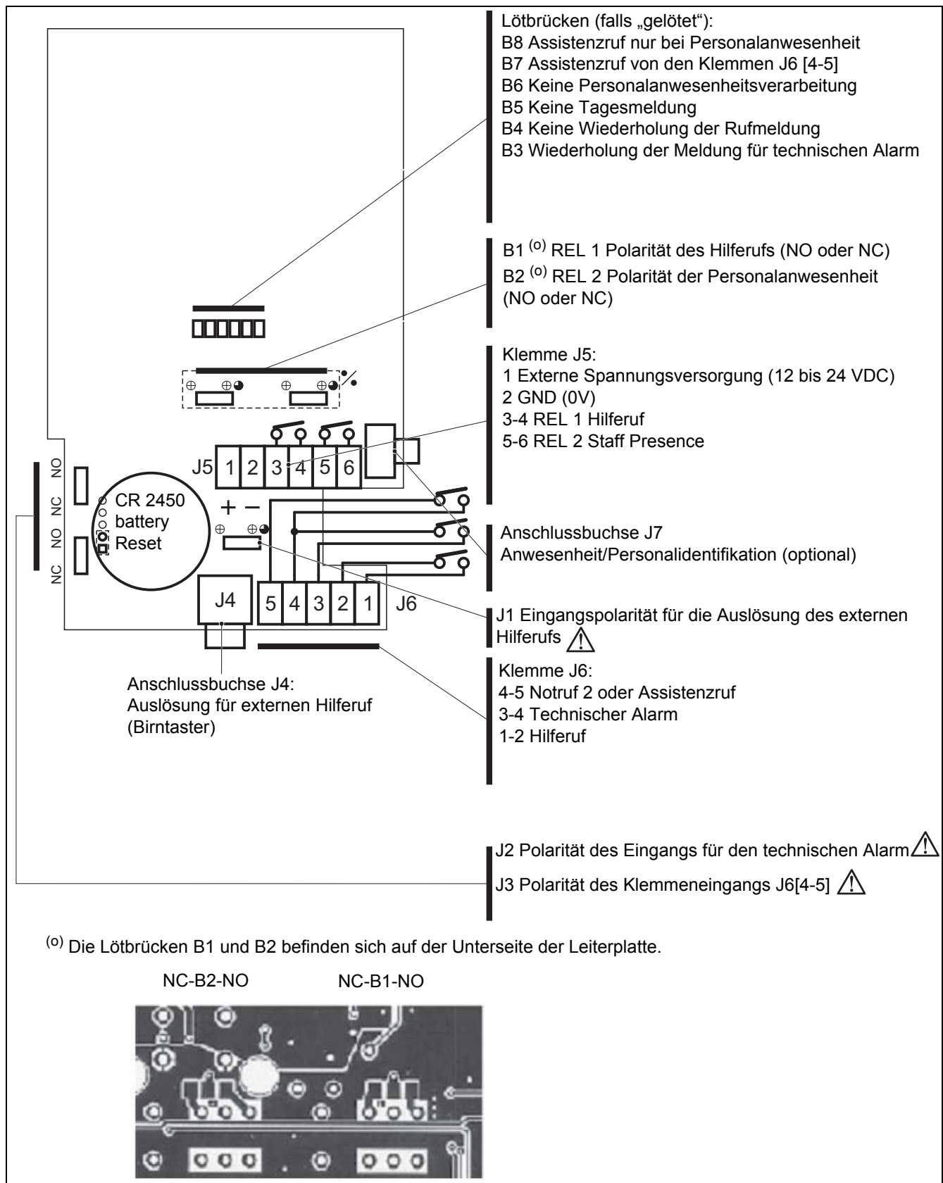
Abb. 5-2: Konfiguration und Anschlussbelegung
